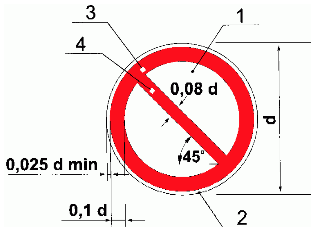
d - диаметр круга; 1 - основная поверхность; 2 - кант; 3 - кайма; 4 - поперечная полоса
