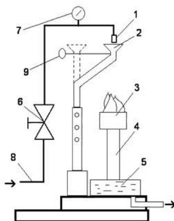
Рис. 1. Схема испытательного стенда:
