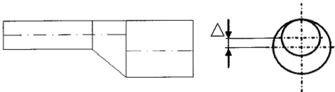
Устройство несоосного перехода труб
